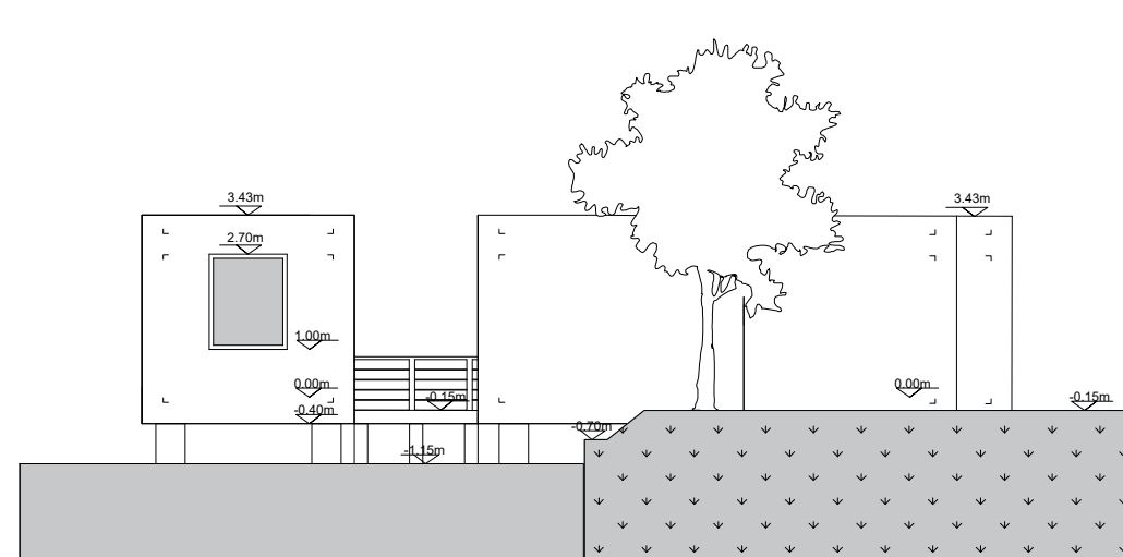
Noordgevel
