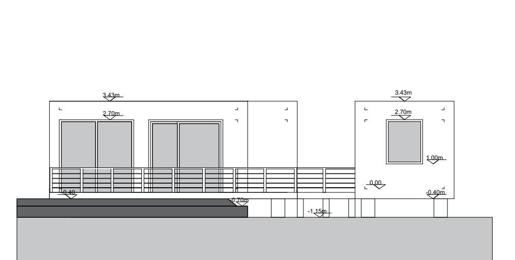
Zuidgevel
