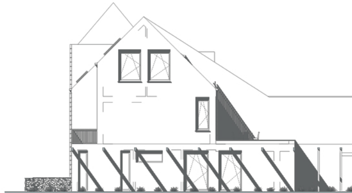
Rechtergevel
