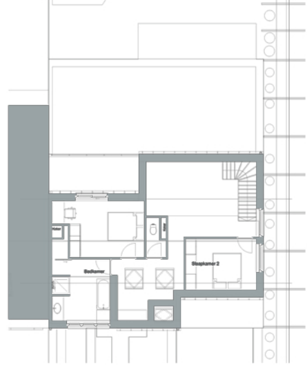
Tweede verdiep
