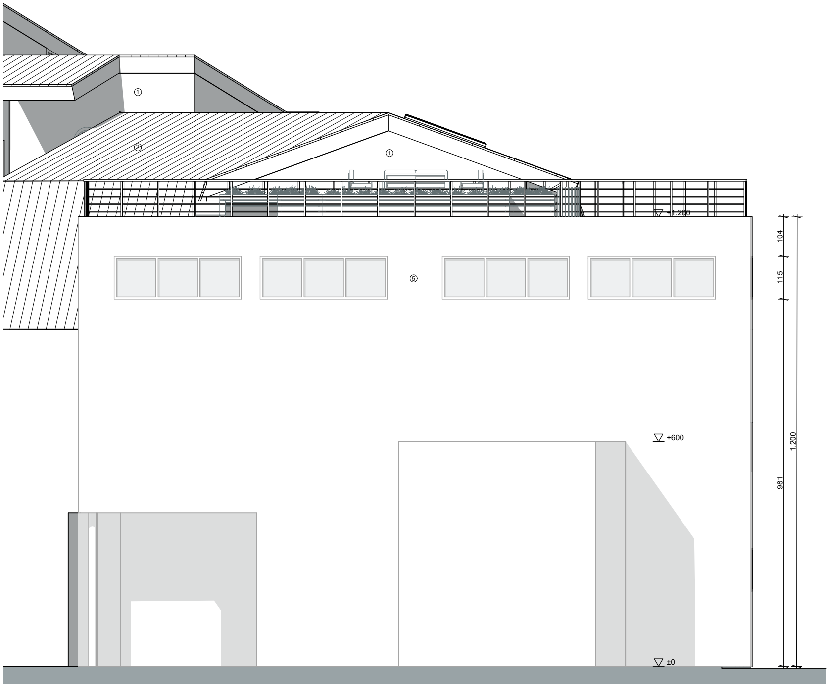
Linkergevel - Noordoosten
