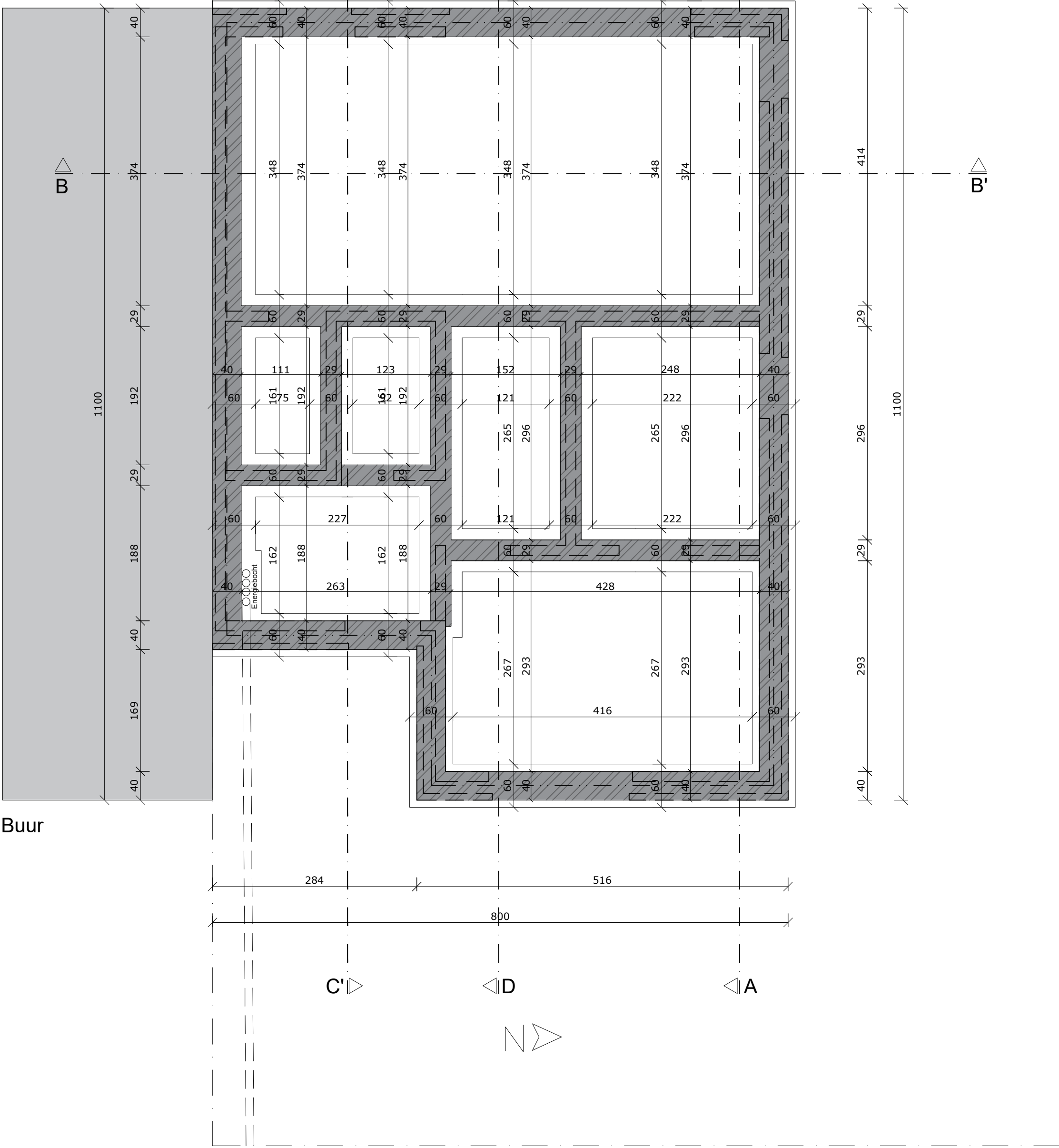
Funderingsplan Schaal 1/50
