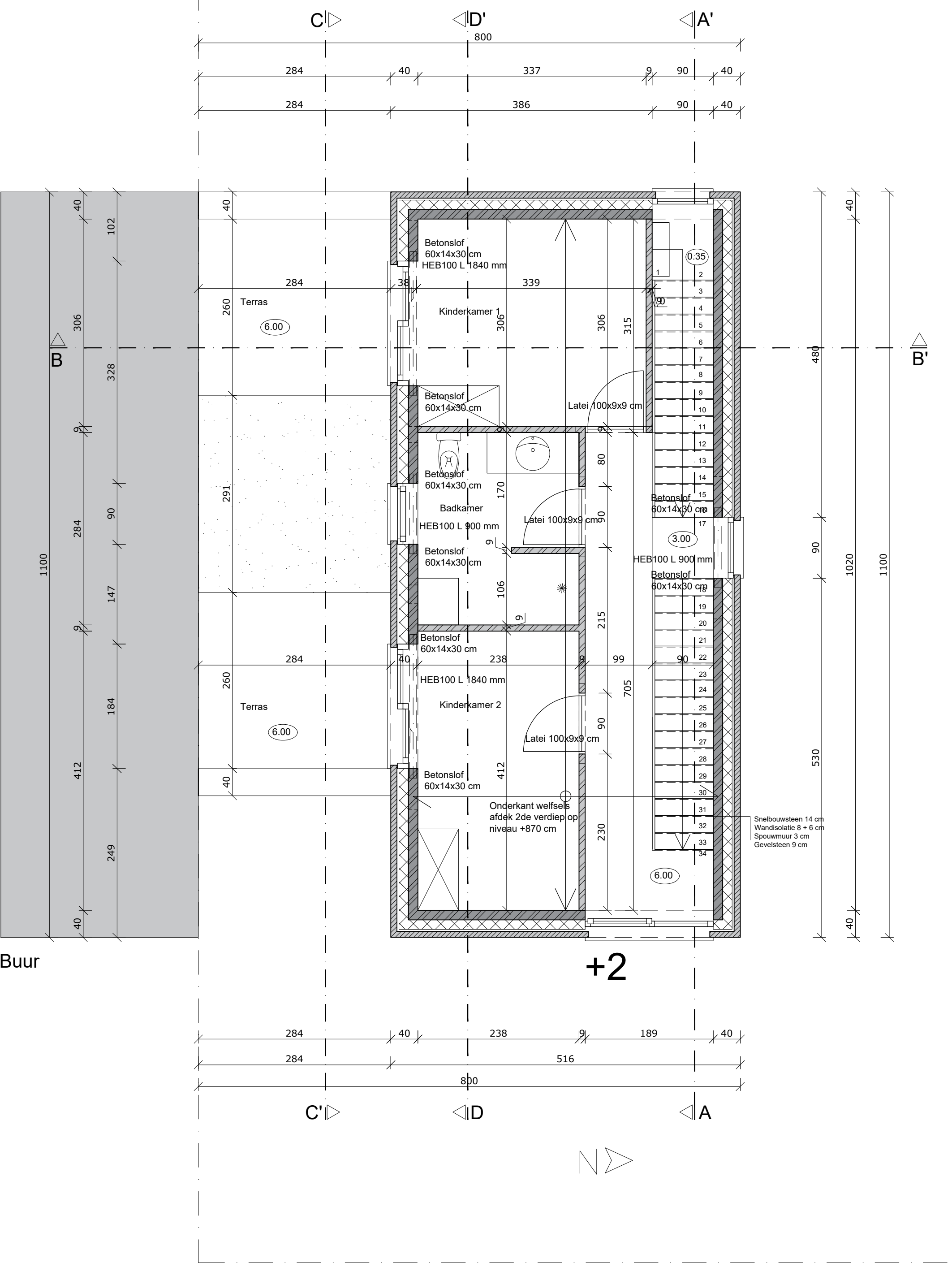
2de verdieping Schaal 1/50
