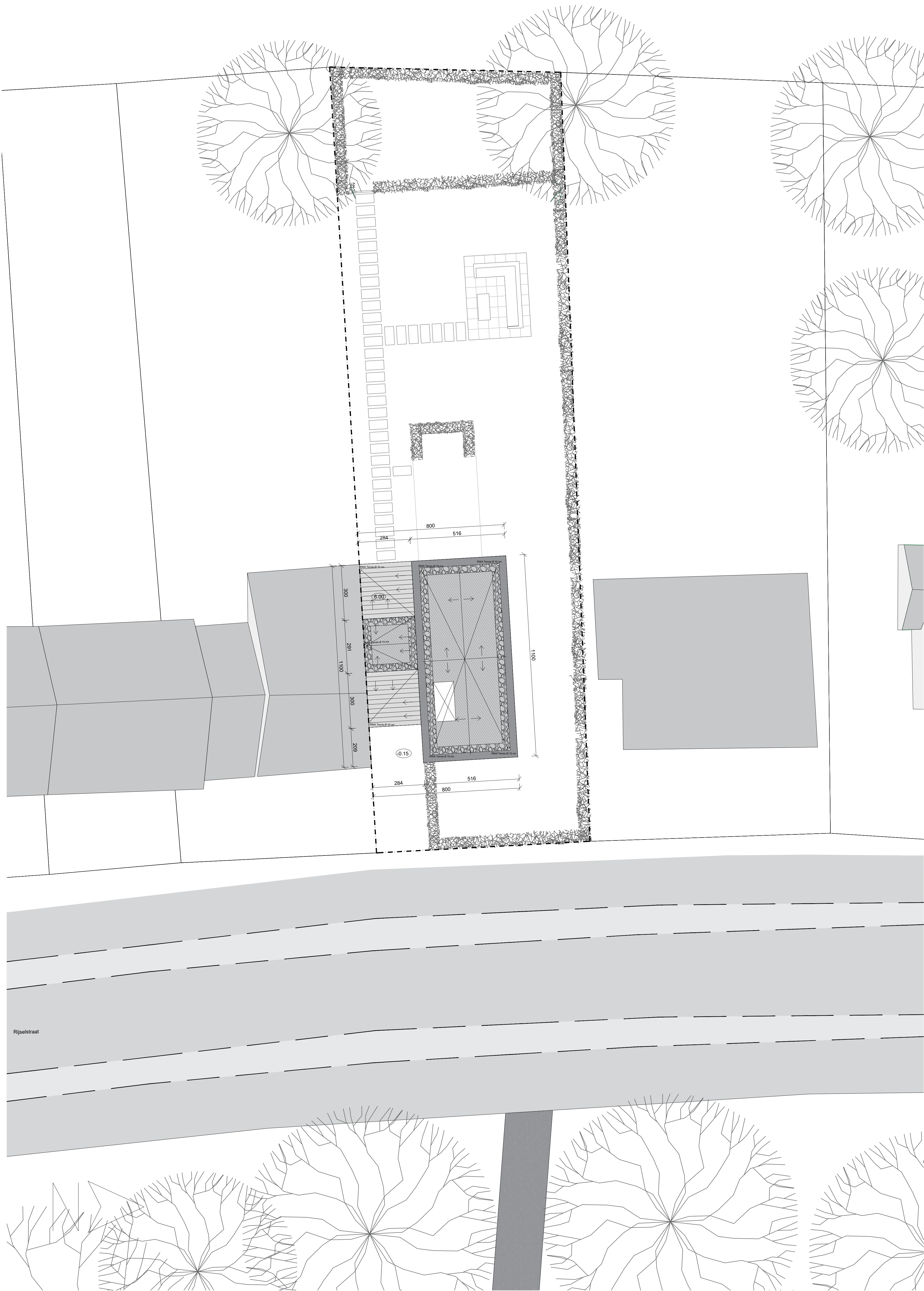
Inplantingsplan Schaal 1/100
