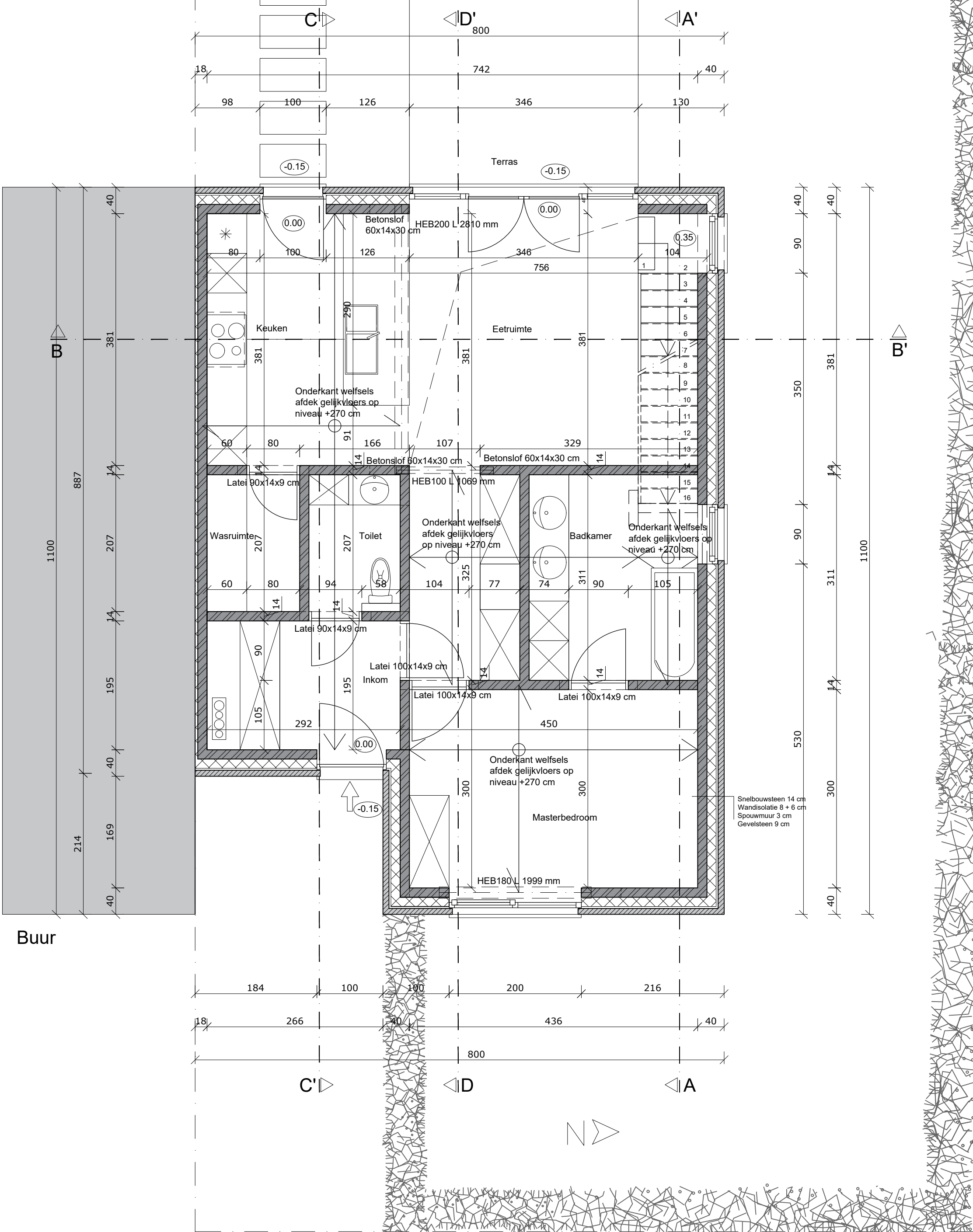
Gelijkvloer Schaal 1/50
