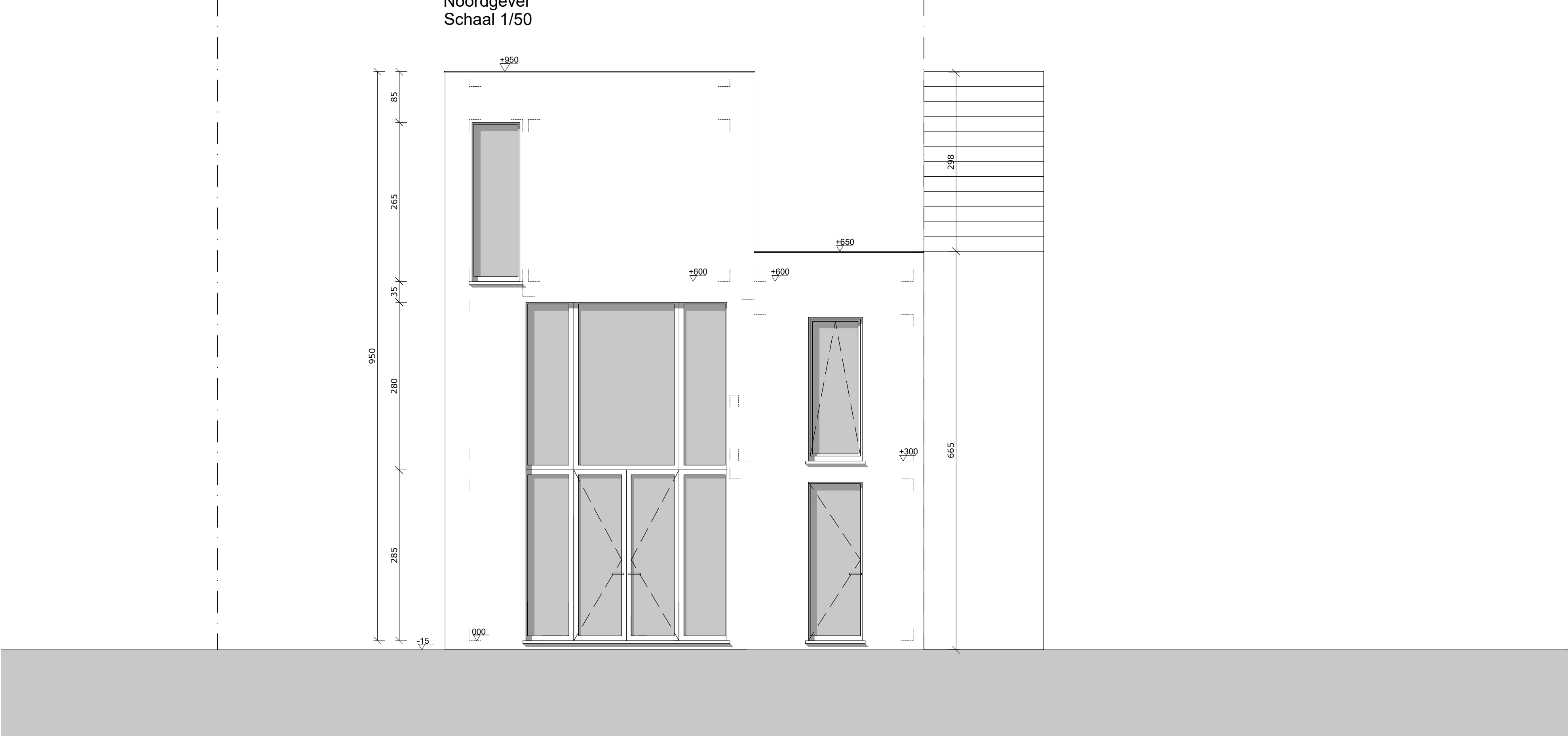
Westgevel Schaal 1/50
