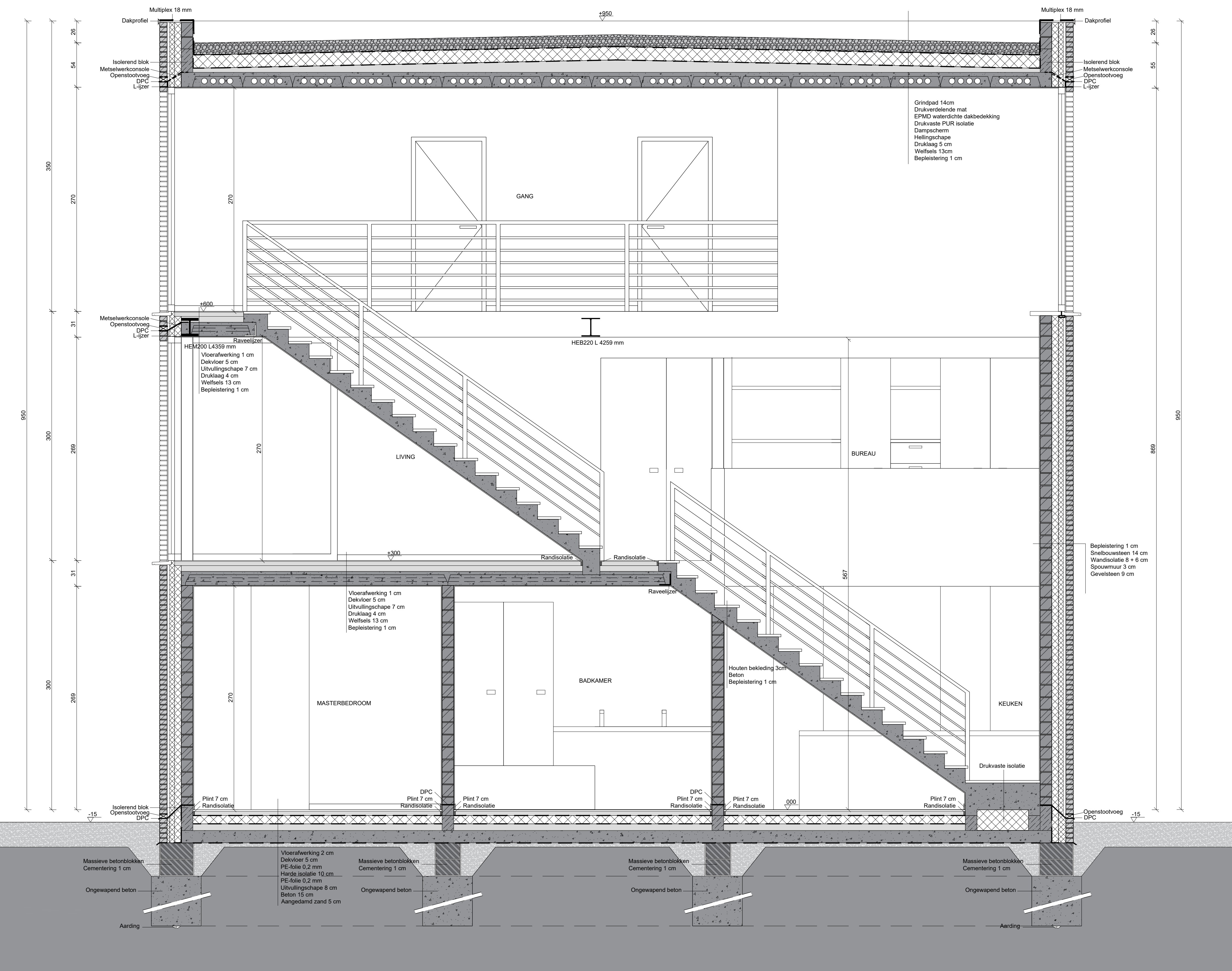
Doorsnede AA' Schaal 1/25
