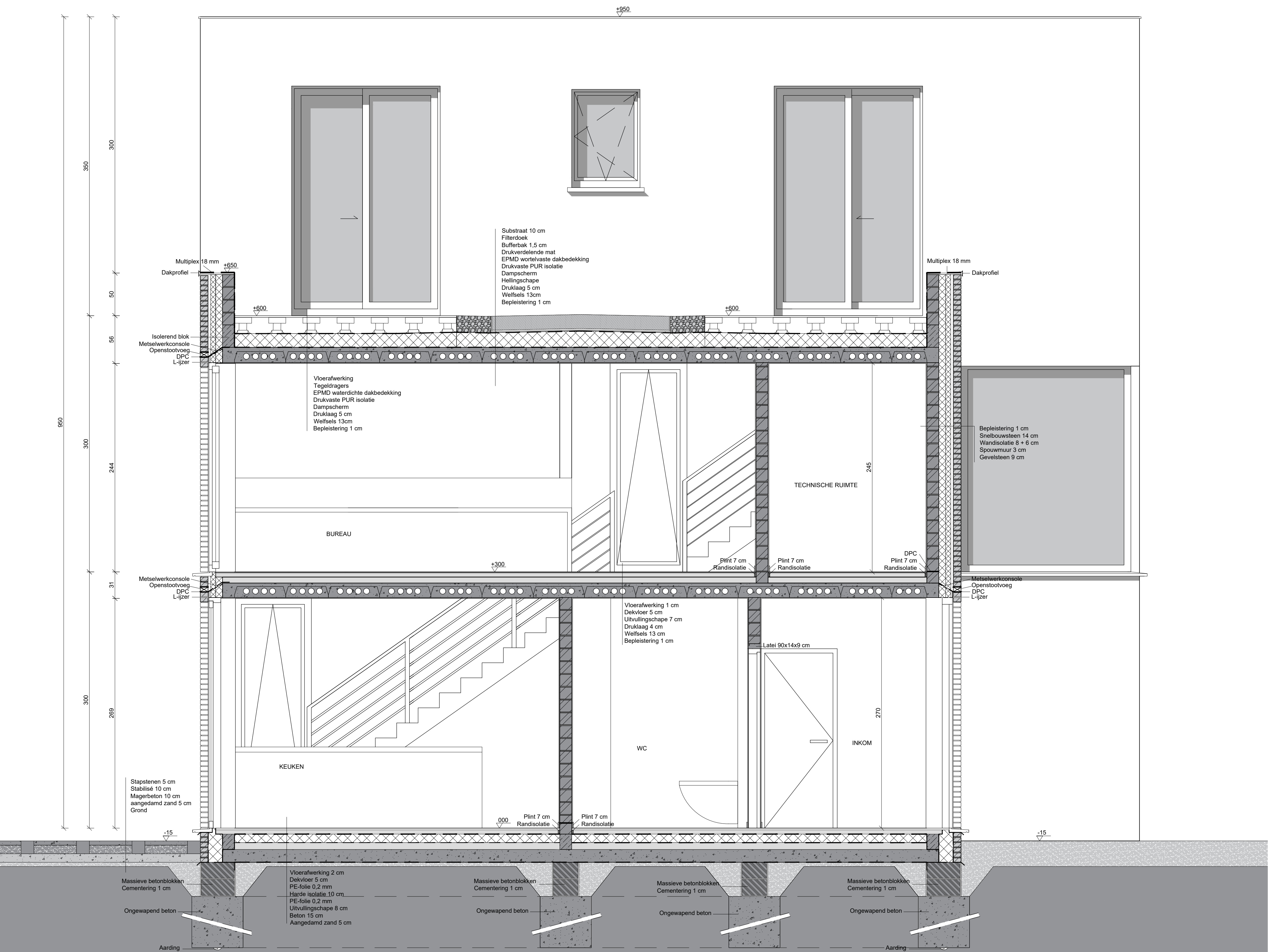
Doorsnede CC' Schaal 1/25
