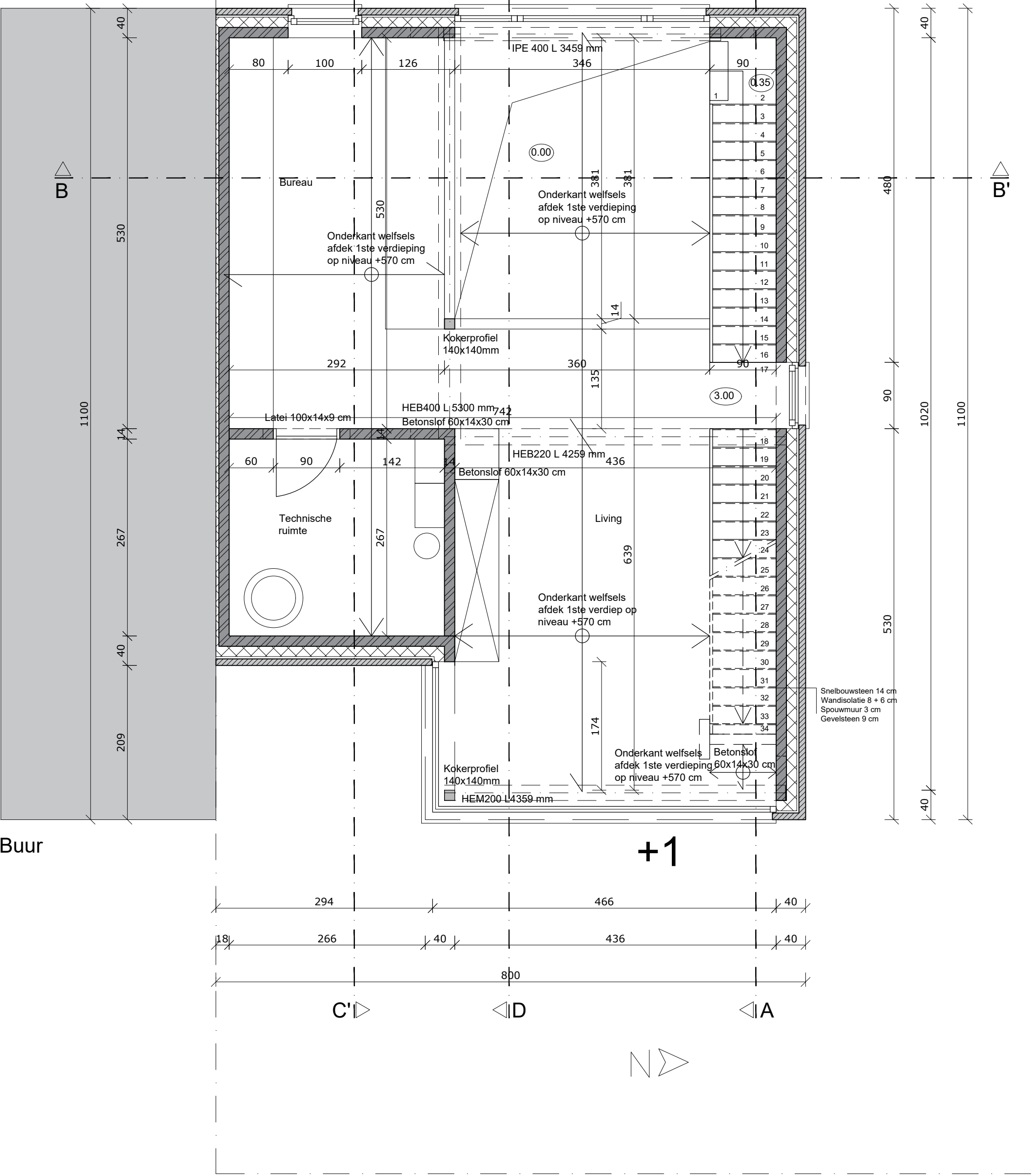
1ste verdieping Schaal 1/50
