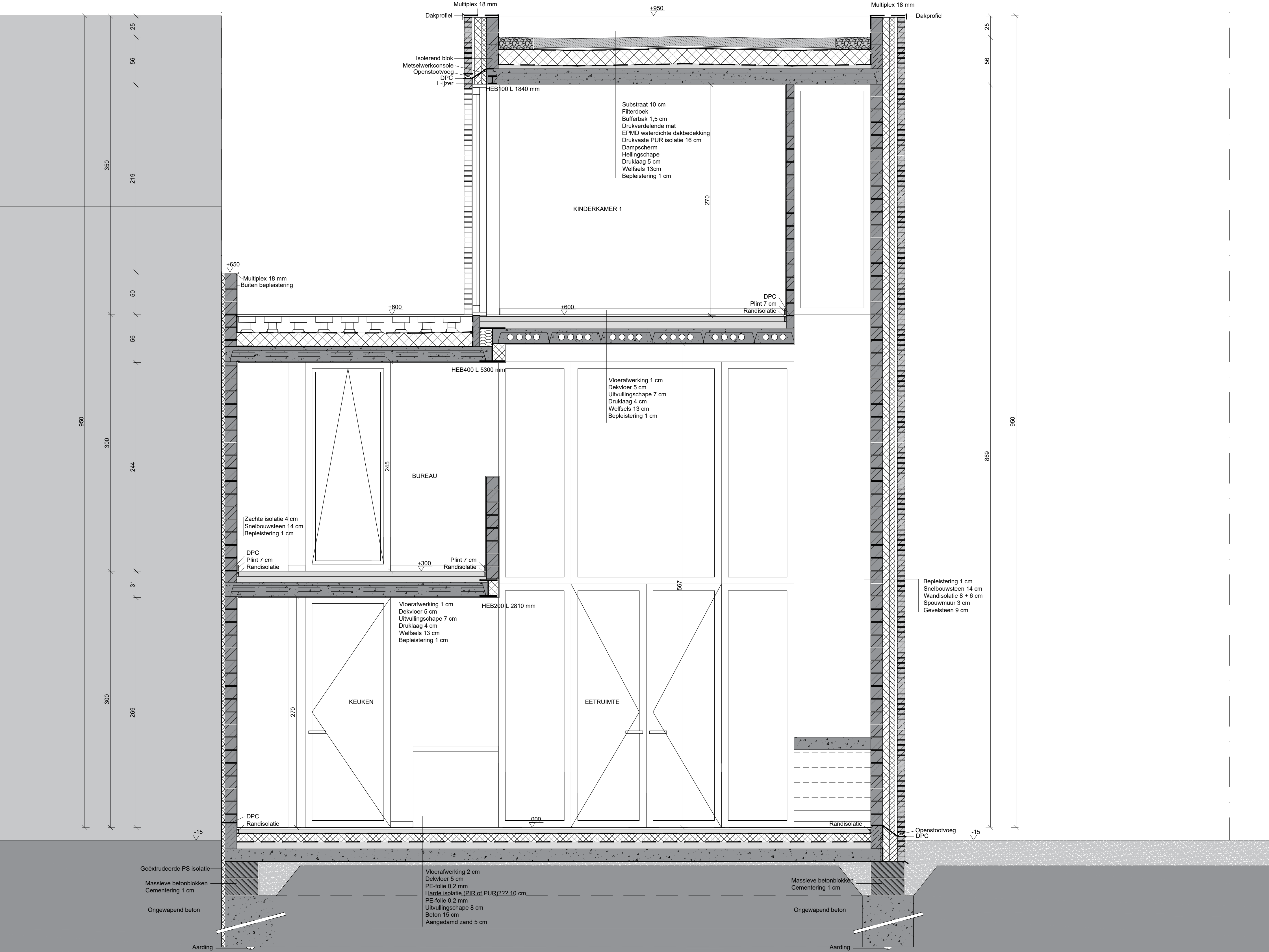
Doorsnede BB' Schaal 1/25
