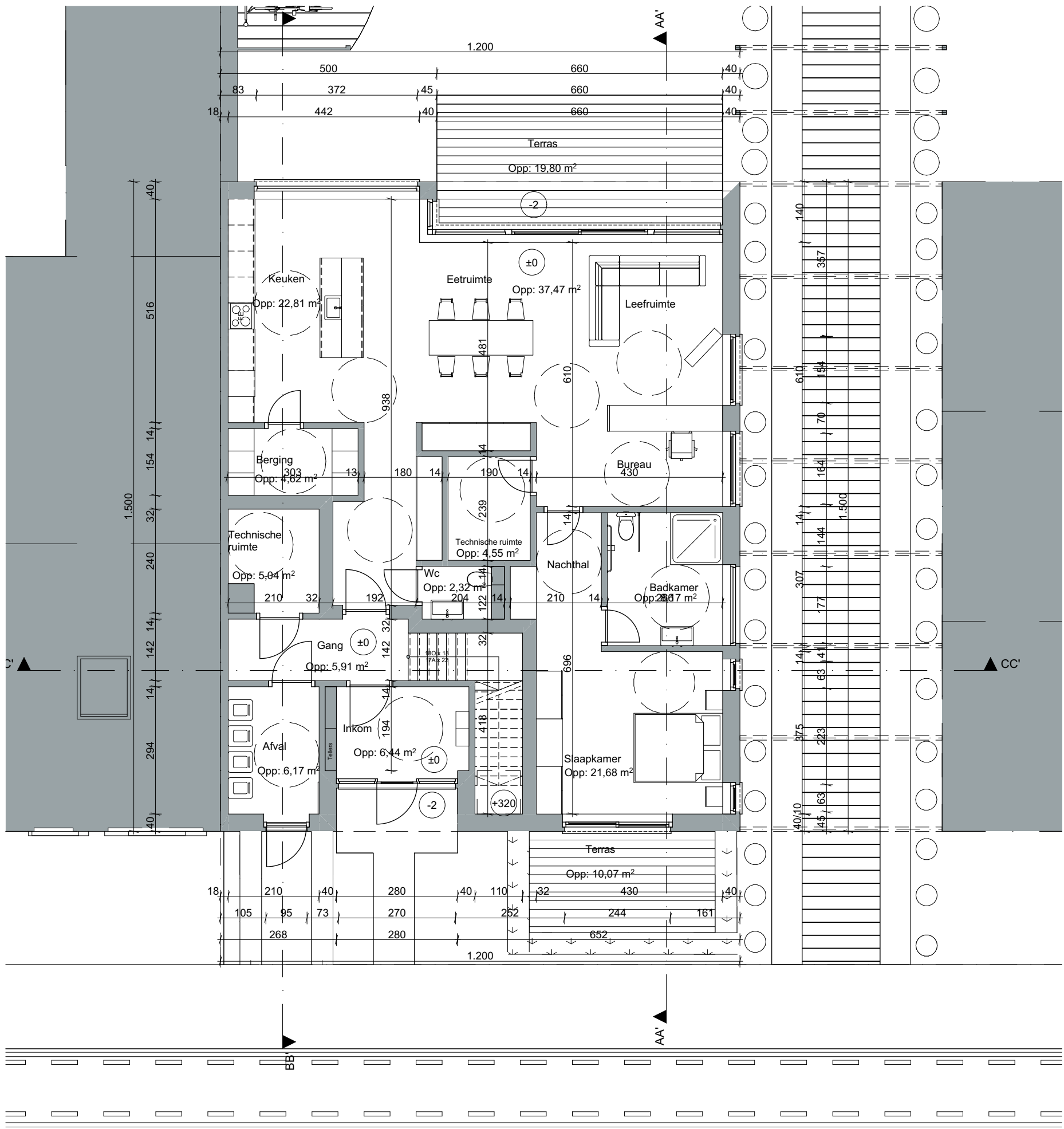
Gelijkvloers
