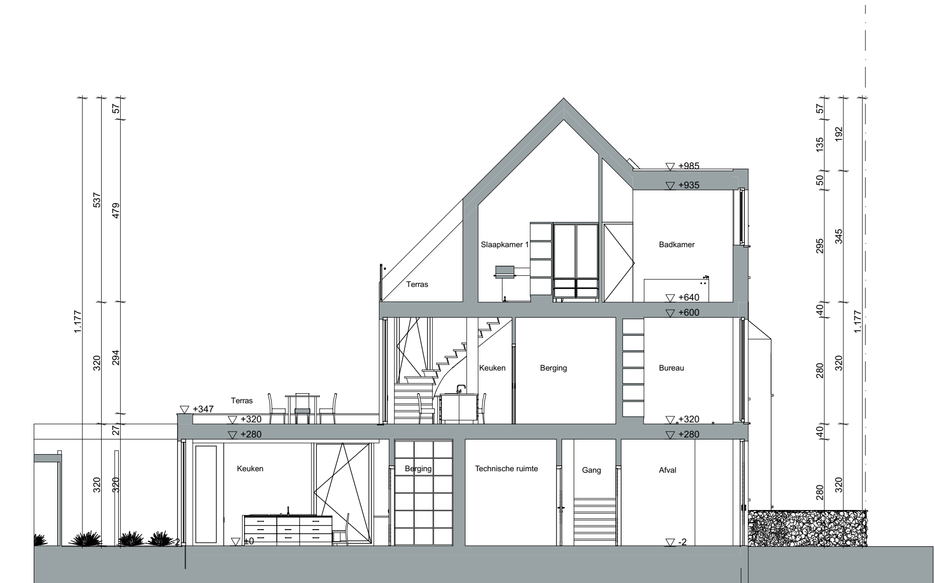
Doorsnede
