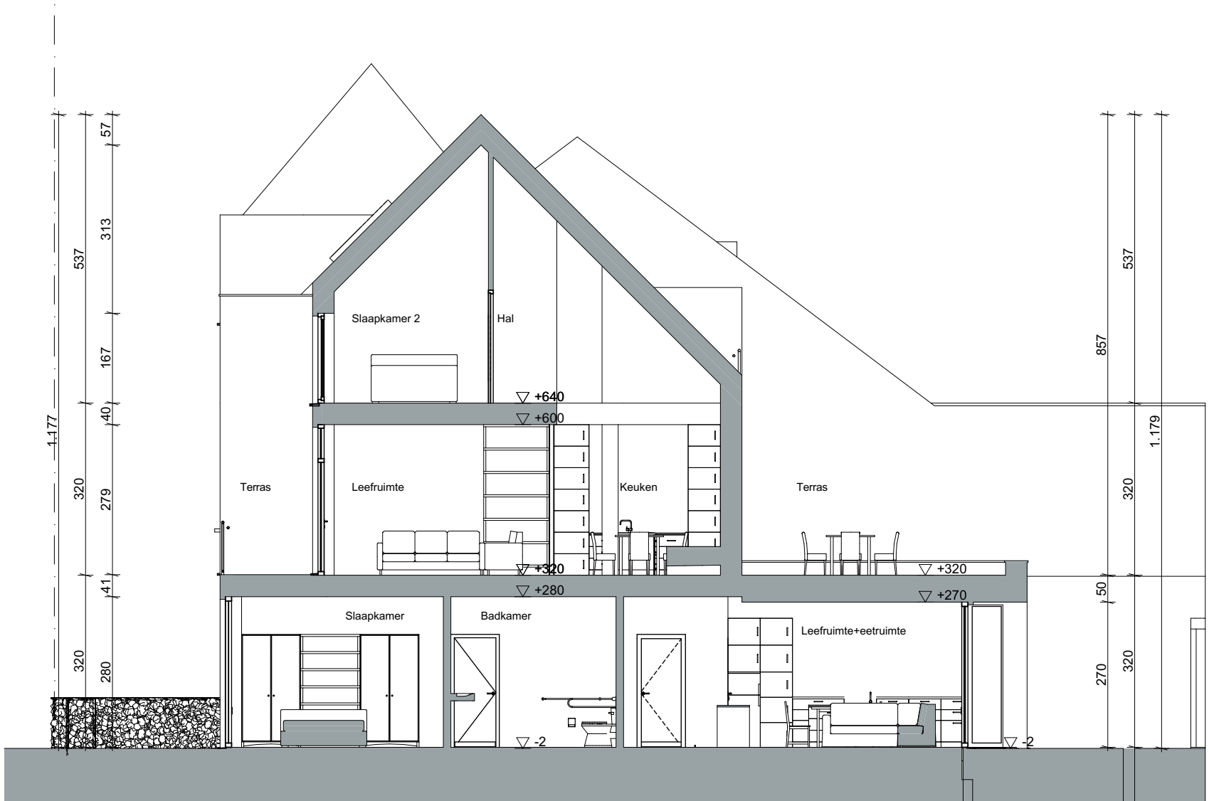
Doorsnede
