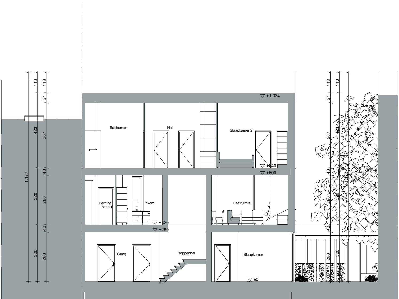
Doorsnede
